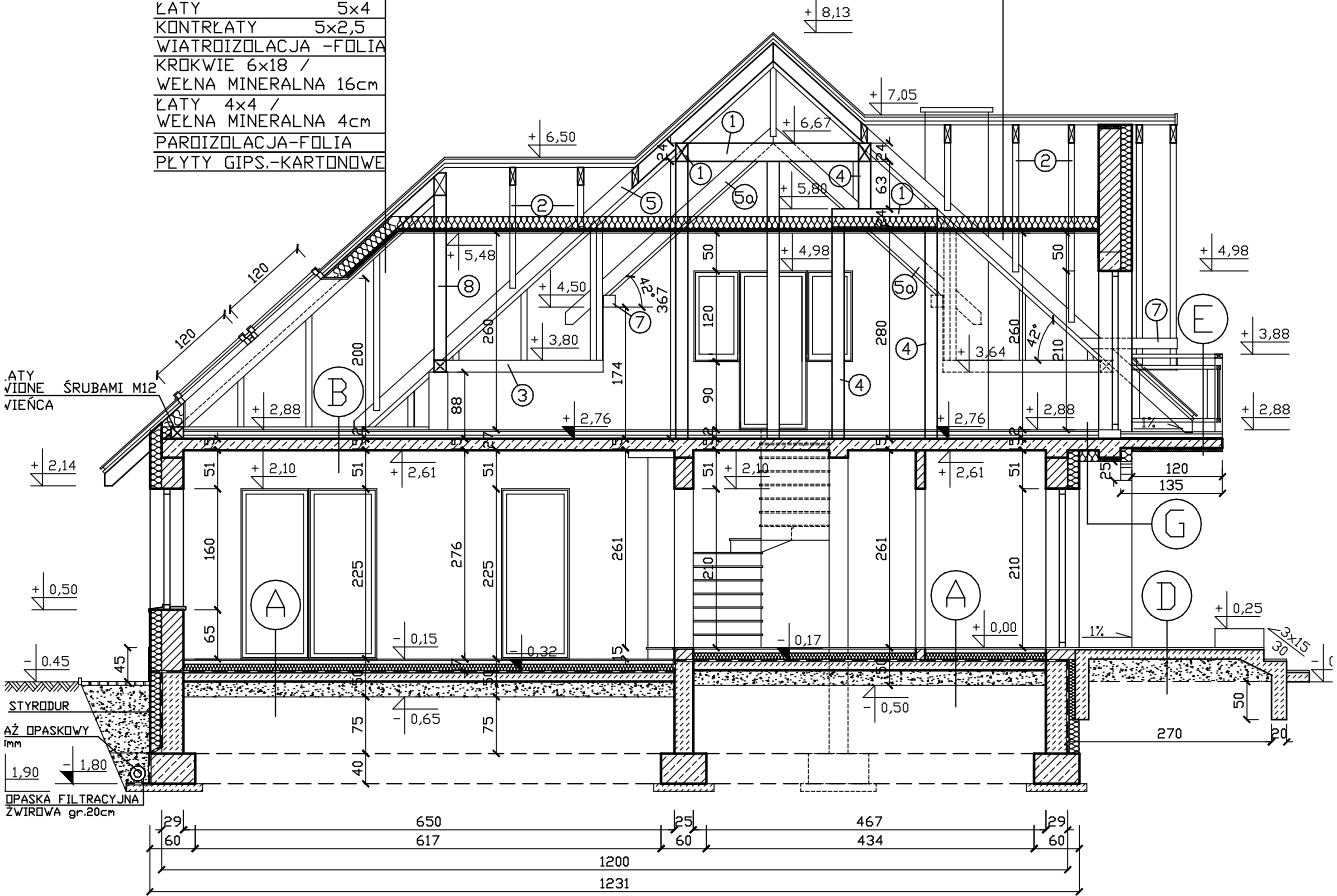
ELEMENTY KONSTRUKCYJNE
